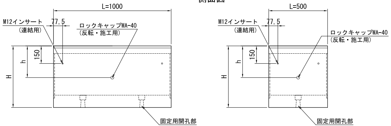
側面図
