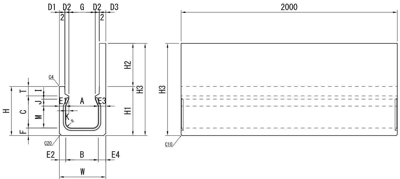
断面図
