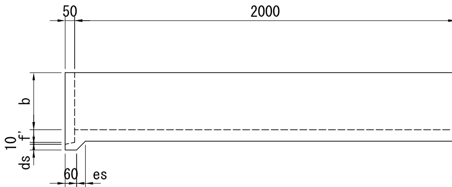
断面図
