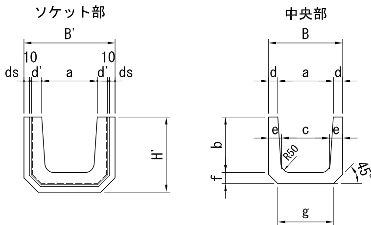
断面図
