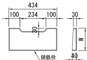
ふた(装鉄製)
