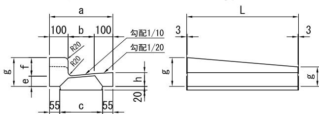
ふた(装鉄製)
