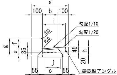
縁塊 断面図
