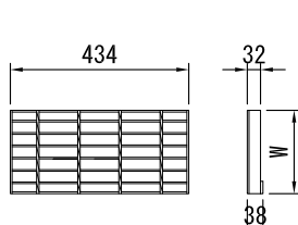
ふた(グレーチング)
