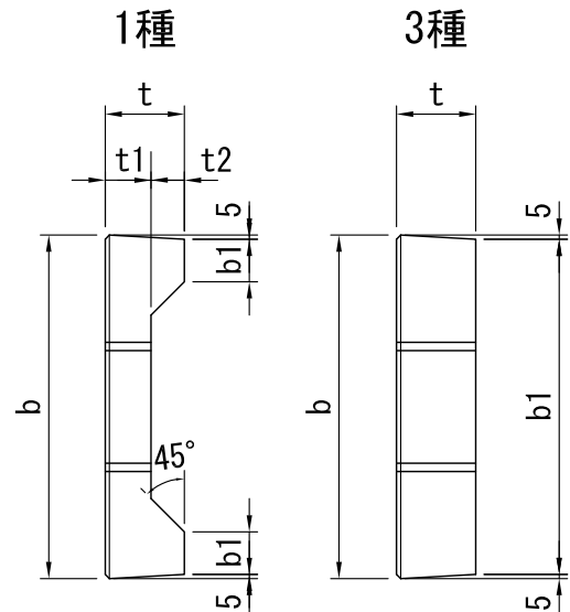
断面図
