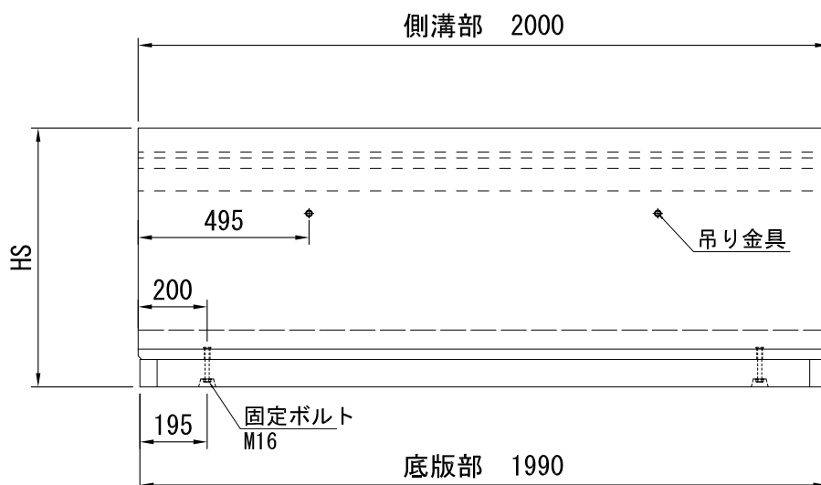
側面図
