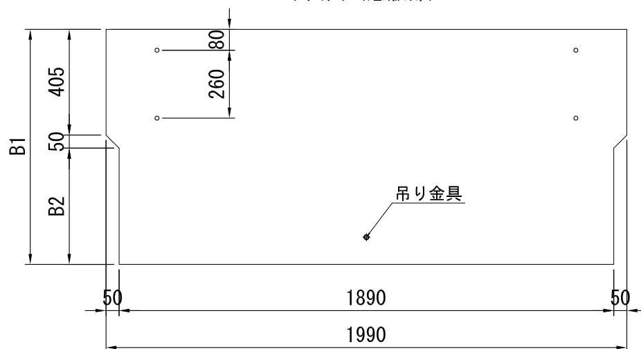
平面図（底版部）
