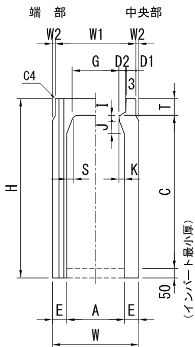
形状図
