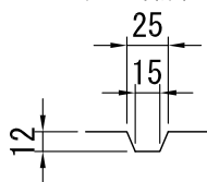
目地部詳細
