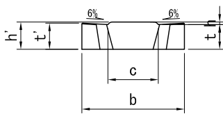
切下げ部 BFLDブロック
