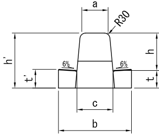
標準部 BFLブロック
