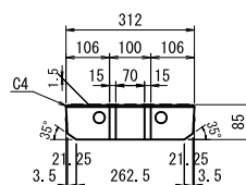
車道用 300用 参考質量 31kg
