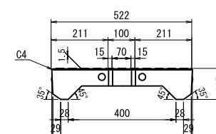
歩道用 500用 参考質量 49kg
