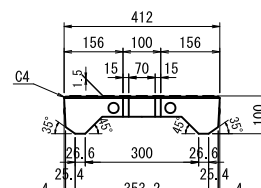
歩道用 400用 参考質量 34kg
