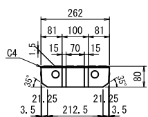
車道用 250用 参考質量 24kg
