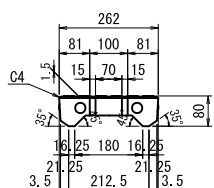
歩道用 250用 参考質量 18kg
