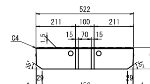
車道用 500用 参考質量 70kg
