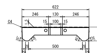
歩道用 600用 参考質量 59kg
