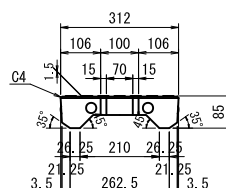
歩道用 300用 参考質量 24kg
