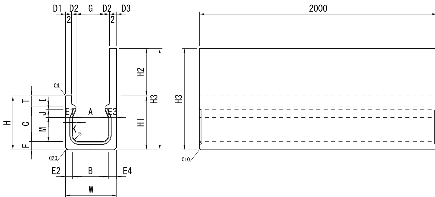
断面図
