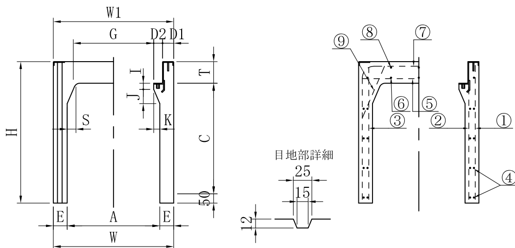
平面図
