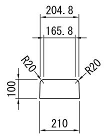
断面図 (C-C)
