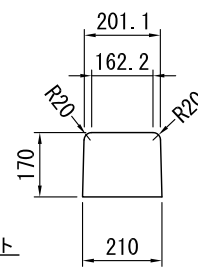
断面図 (B-B)
