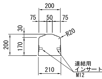
断面図 (A-A)
