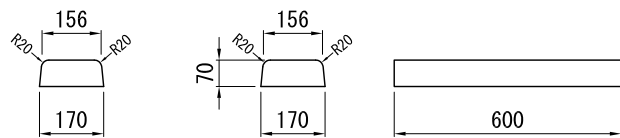
FD-A型切下げ 参考質量 17kg
