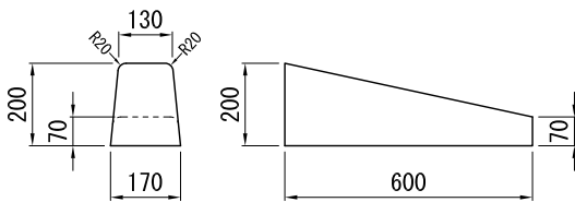
FT-B型1段すり付け 参考質量 47kg
