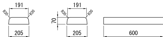
FD-B型切下げ 参考質量 18kg
