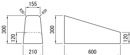
FT-C型1段すり付け 参考質量 56kg
