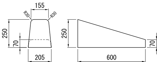
FT-C型1段すり付け 参考質量 56kg
