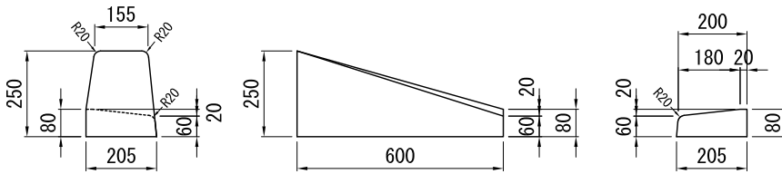
FS-B/MD-B0改 1段すり付け 参考質量 43kg
