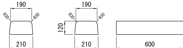
FD-C型切下げ 参考質量 33kg
