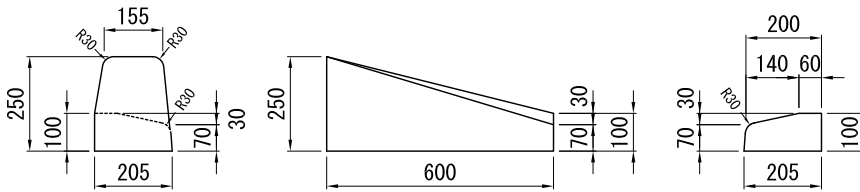
FS-B/MD-B1 1段すり付け 参考質量 46kg
