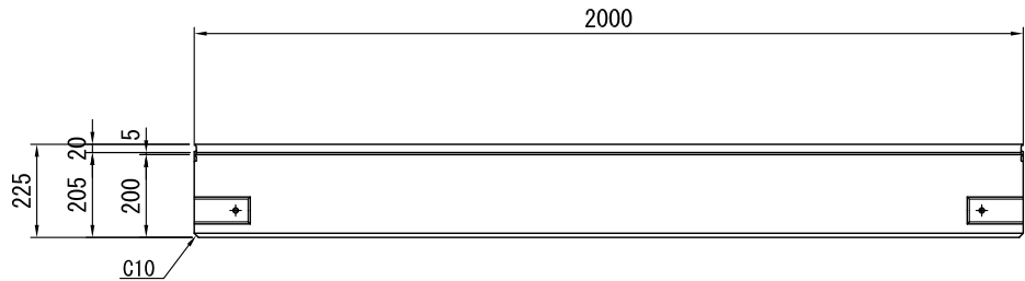
側面図
