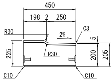
断面図
