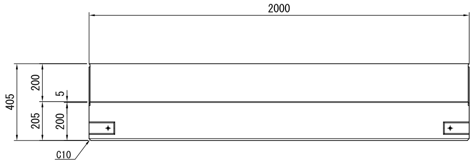
平面図
