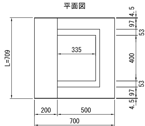
グレーチング
