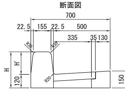
CBL2標準型縁塊
