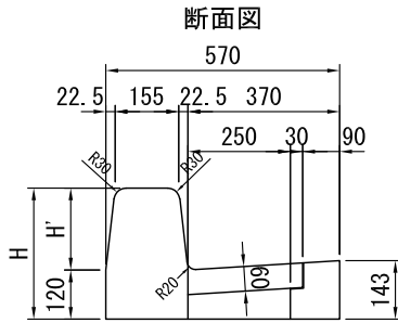
CBL1標準型縁塊
