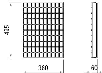
グレーチング
