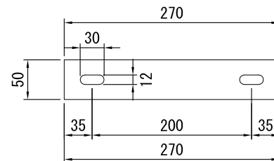
連結用プレート (M10用) 厚さ 3.0mm
