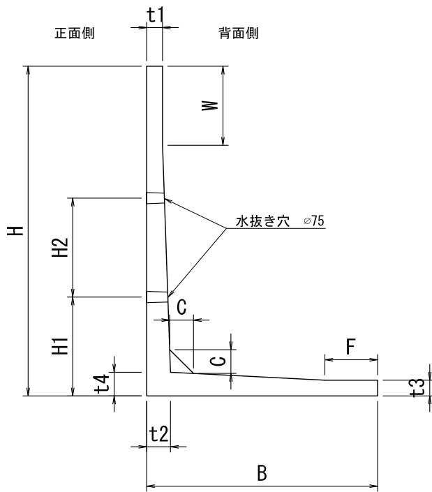
断面図
