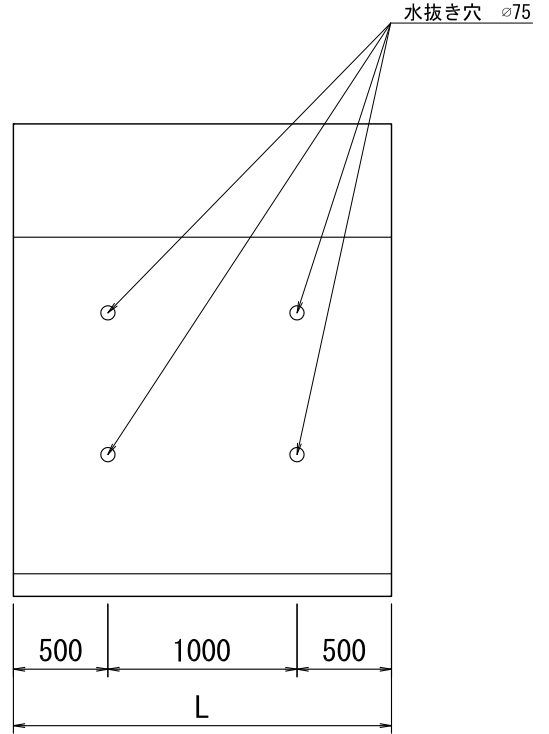
側面図（背面）
